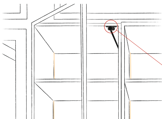
Ref: 41.121 Interruptor con sensor para puerta o cajón 12V - 24V / Sensor switch for door or drawer 12V - 24V
