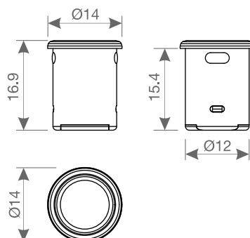
Ref: 41.123 Interruptor con sensor doble para puertas o cajones 12V - 24V / Dual sensor switch for doors or drawers 12V - 24V
