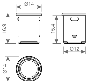
Ref: 41.121 Interruptor con sensor para puerta o cajón 12V - 24V / Sensor switch for door or drawer 12V - 24V
